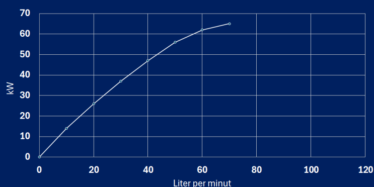
90° C - Køleeffekt
